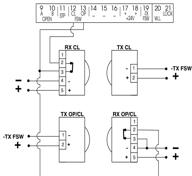
Conexión de una pareja de fotocélulas en cierre y otra en apertura/cierre (esquema aconsejado)
