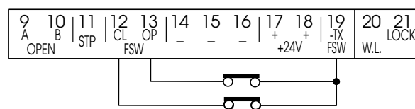
Conexión de un dispositivo de seguridad en cierre y de un dispositivo de seguridad en apertura
