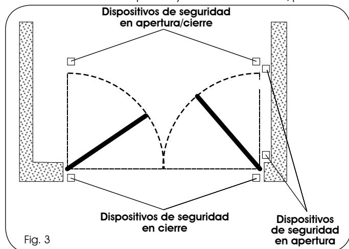
Conexión de una pareja de fotocélulas en cierre, una en apertura y una en apertura/cierre (esquema aconsejado)
