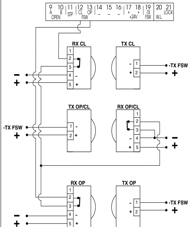
Conexión de una pareja de fotocélulas en cierre, una en apertura y una en apertura/cierre (esquema aconsejado)
