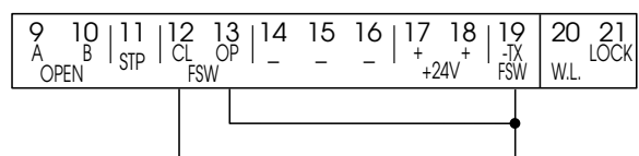
Conexión de ningún dispositivo de seguridad
