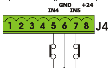
Conexión de un dispositivo de seguridad en cierre y de un dispositivo de seguridad en apertura
