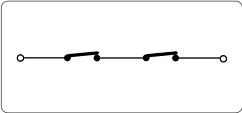
Fig. Conexión de 2 contactos N.C. en serie.
