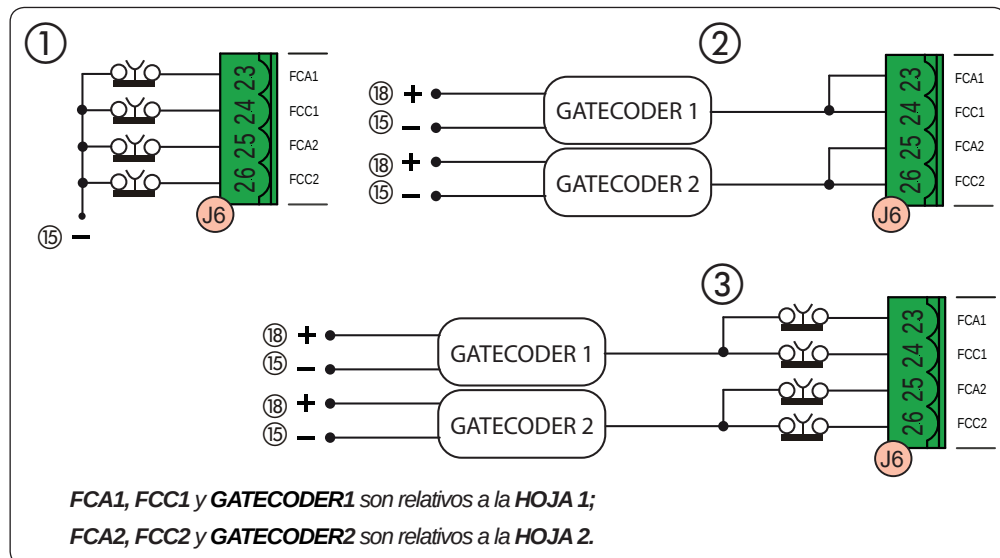
Fig. Conexiones de los finales de carrera y GATECODER (máxima configuración: ③).
