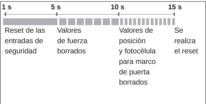
Fig. Sinopsis de la secuencia de tiempo del LED de estado (Status) en el carro al accionar el pulsador Reset verde
